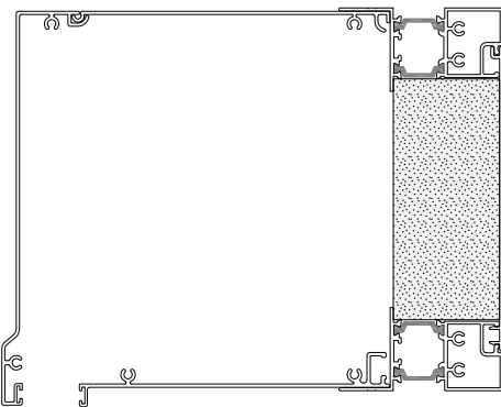
Γ. Ίσιο κουτί ρολού θερμοδιακοπής
