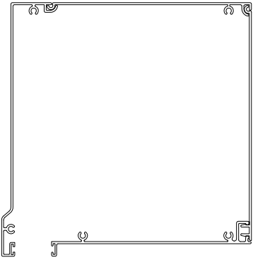
A. Ίσιο κουτί ρολού
