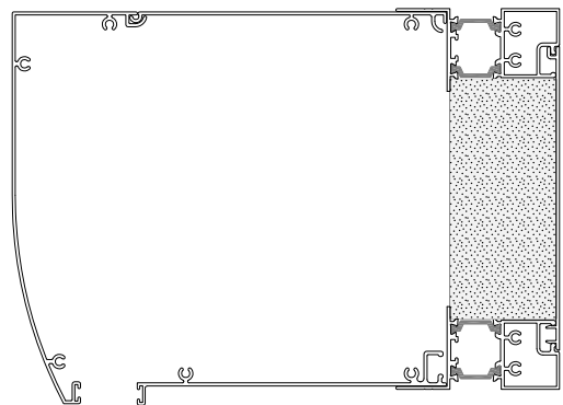
Δ. Οβάλ κουτί ρολού θερμοδιακοπής
