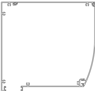
Ε. Εξωτερικό οβάλ κουτί ρολού
