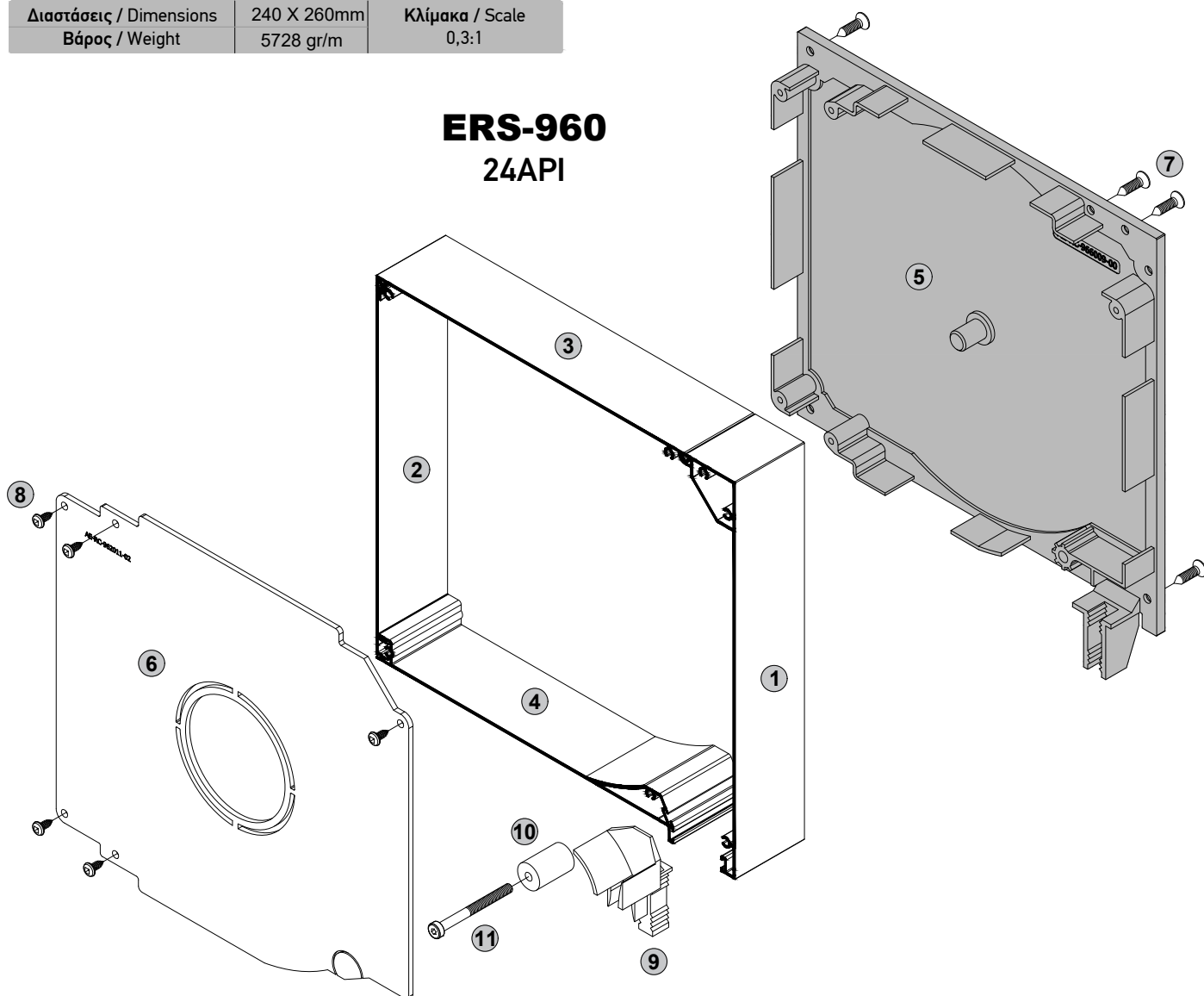
Βασικά Εξαρτήματα Κουτιού (240mm X 260mm)/ Main Parts for Shutter Box (240mm X 260mm)
