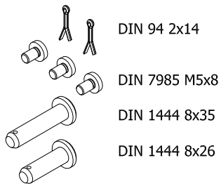
Εξαρτήματα Σύνδεσης Μοτέρ
