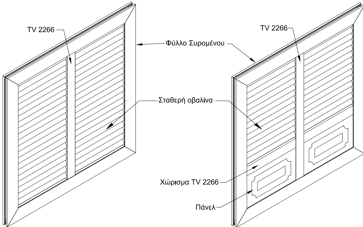
A. Φύλλο συρομένου πατζουριού με κάθετο προφίλ διαχωρισμού.
