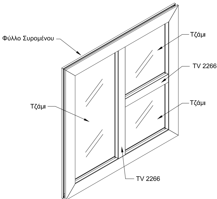
Γ. Φύλλο συρομένου τζαμιού με κάθετο και οριζόντιο προφίλ διαχωρισμού.
