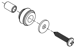
Ράουλο Κρυφής Σήτας Roller for Hidden Insect Screen
