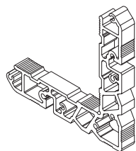
Γωνία Συνδέσεως/Γωνιάστρας του TH 80115 Corner Joint/Crimping for TH 80115
