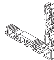
Γωνία Συνδέσεως/Γωνιάστρας του TH 80109 Corner Joint/Crimping for TH 80109
