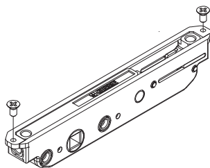
Κλειδαριά Γωνιακής Κατασκευής Lock Mechanism For Corner Structure
